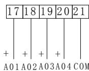
P/Q/I模拟量输出 P/Q/I Analog output
